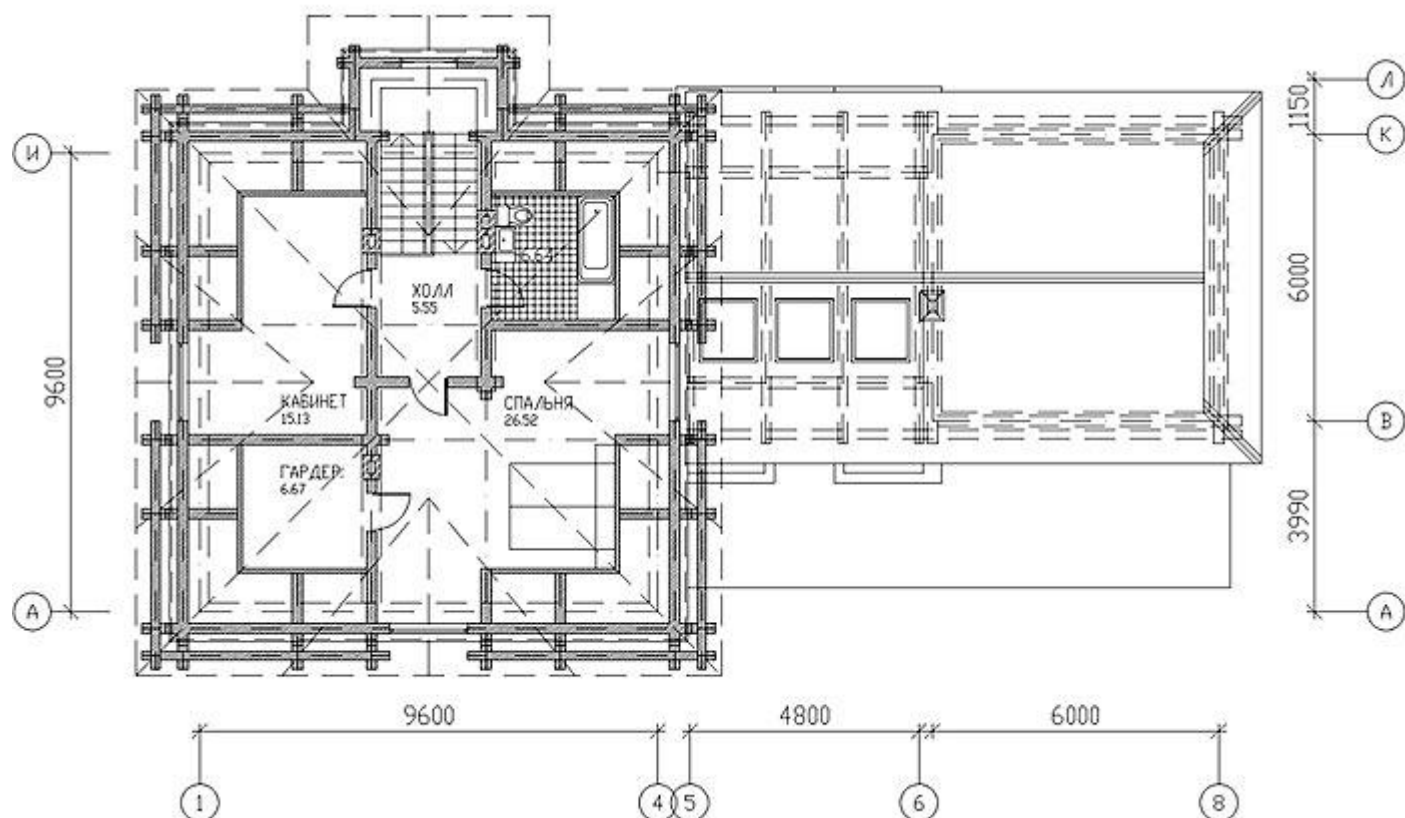
Планировка дома - План 2 этажа
