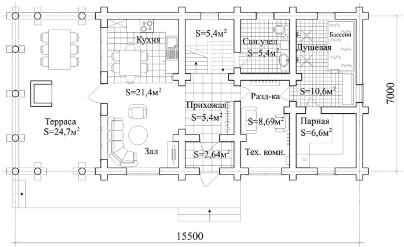
Планировка дома - План 1 этажа высота этажа - 3 м
