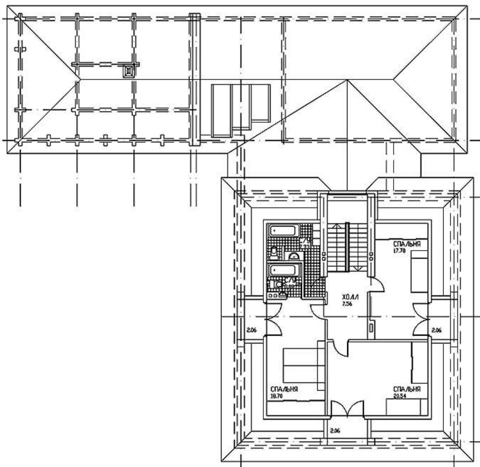
Планировка дома - План 2 этажа
