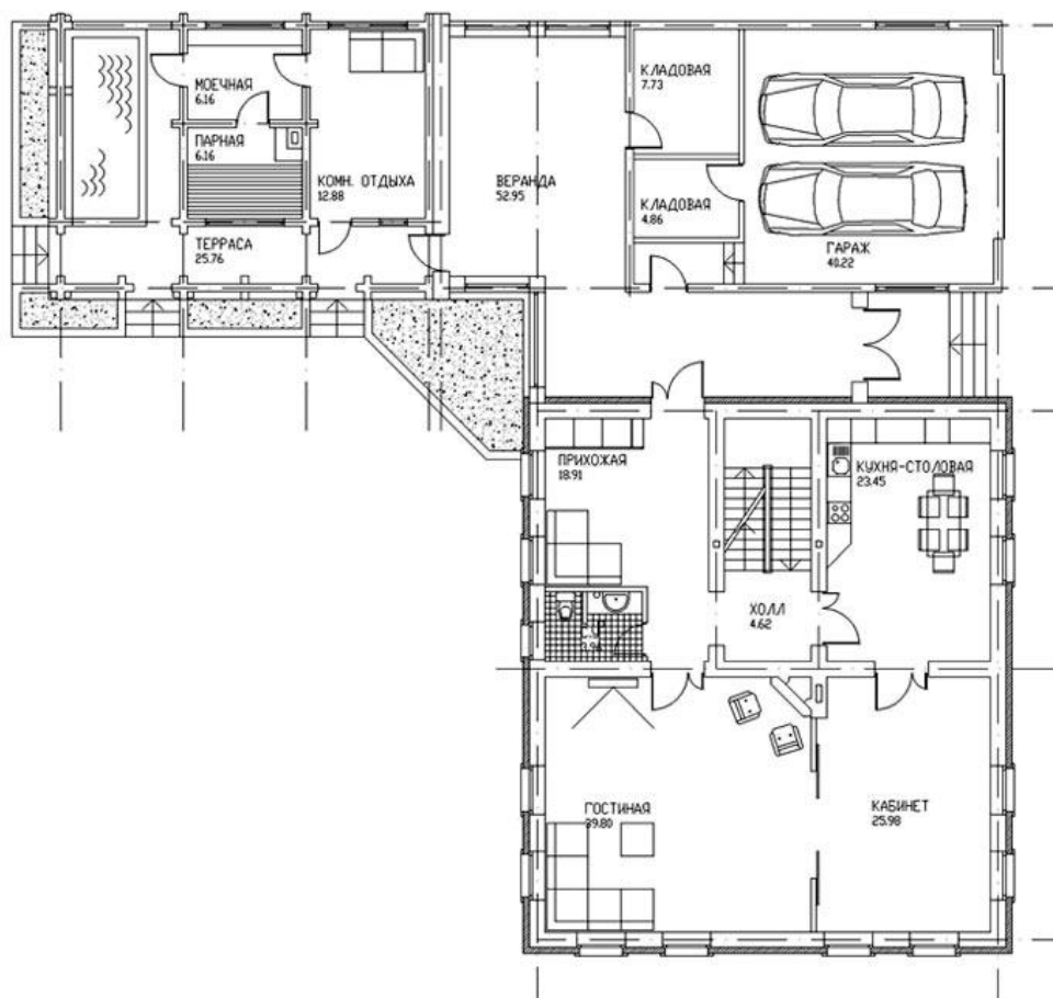
Планировка дома - План 1 этажа
