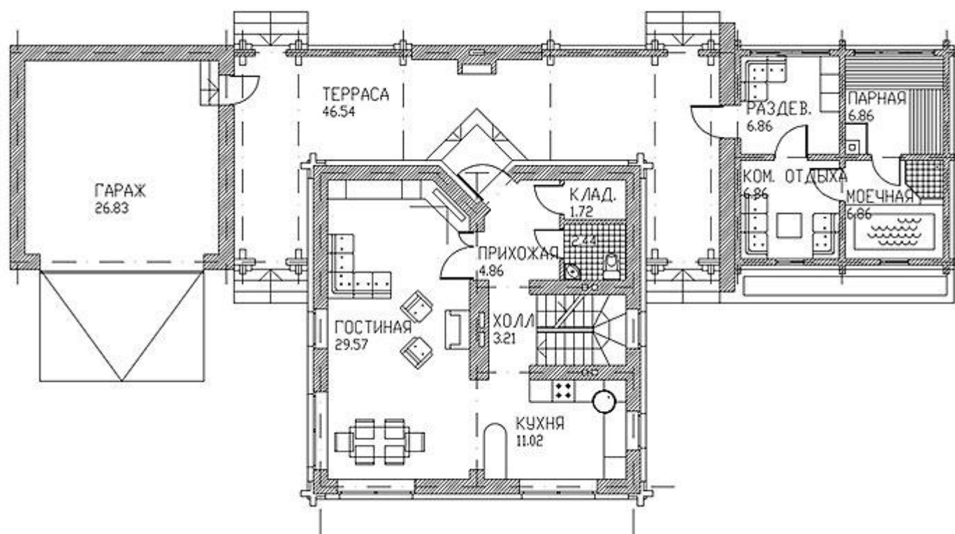
Планировка дома - План 1 этажа
