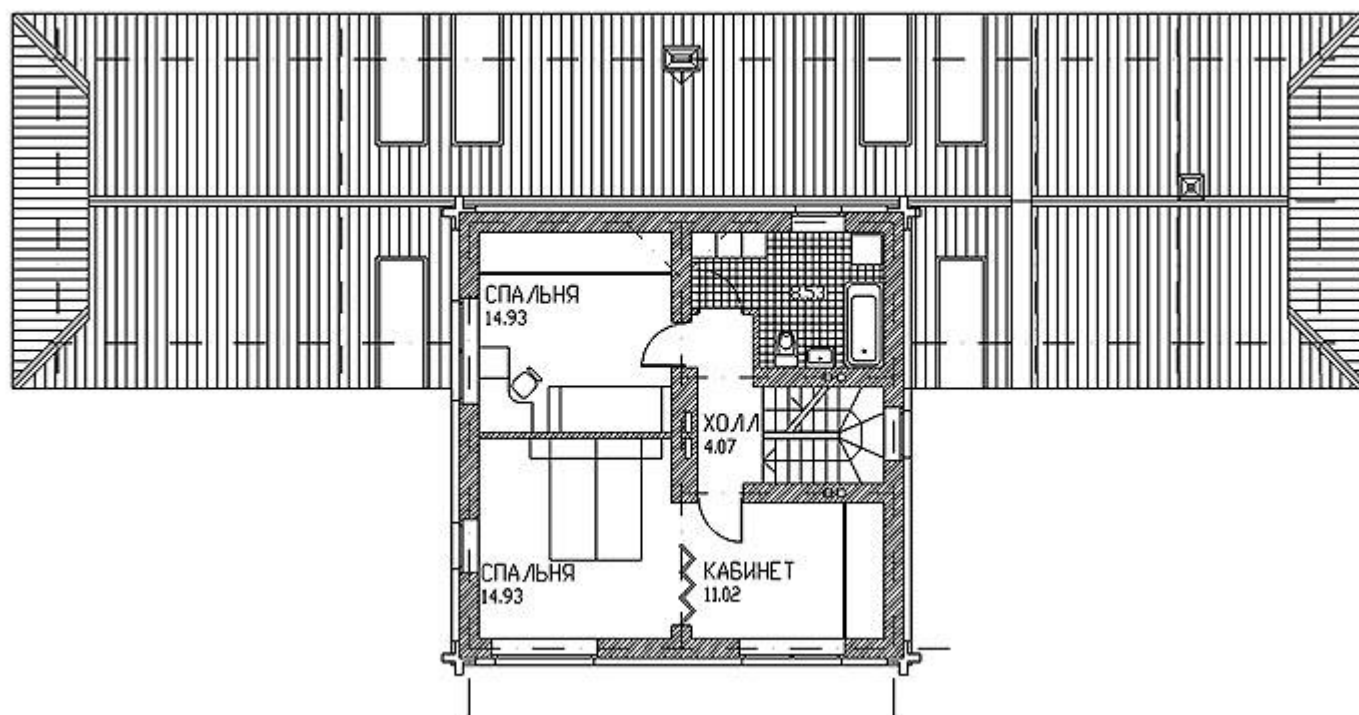
Планировка дома - План 2 этажа
